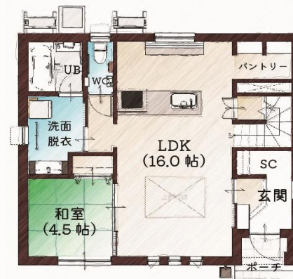
1階平面図
