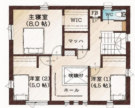
2階平面図
